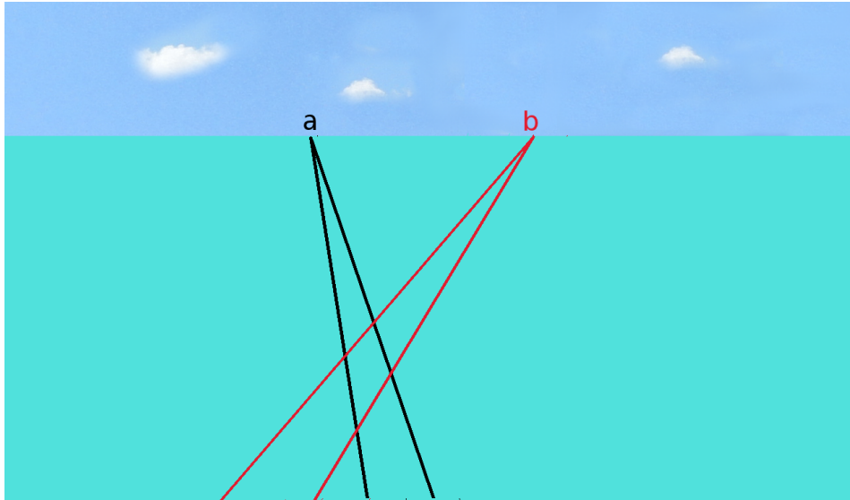
FIGURE 3 – Le plan affine complété par une droite à l’infini
