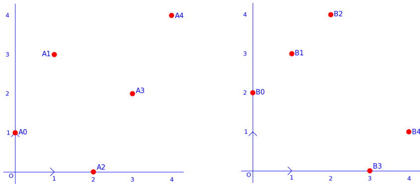
FIGURE 9 – À gauche D_1 , à droite D_2 , de pente 1, passant par B_0 = (0, 2)
