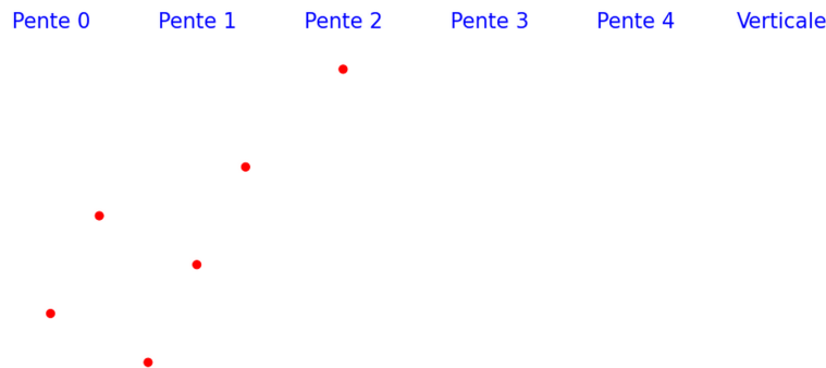
FIGURE 11 – Les 6 points de la droite projective associée à D_1 .
