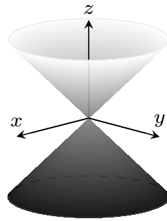
Cône
