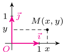
Plan cartésien : (\mathbb{R}^2, (O, \vec{i}, \vec{j}))
