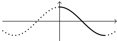
La fonction cosinus restreinte à [0, \pi] est inversible
