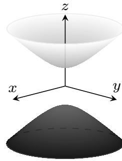
Hyperboloïde à deux nappes
