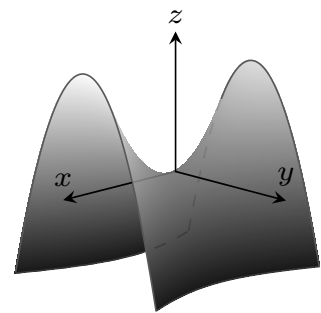
Paraboloïde hyperbolique
