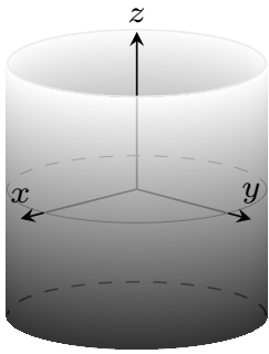
Cylindre
