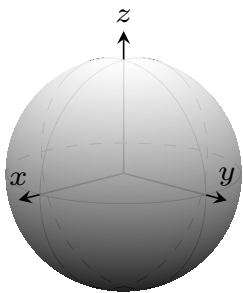
Sphère
