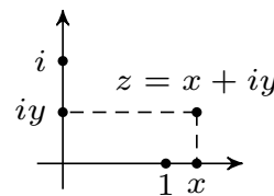
Plan complexe : \mathbb{C}
