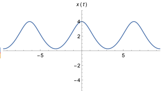
solution de (EC)
