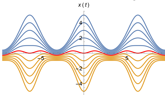
solutions de l'équation complète
