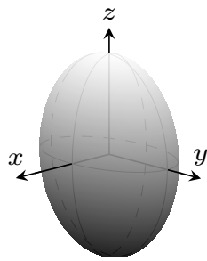
Ellipsoïde
