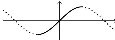
La fonction sinus restreinte à [-\pi/2, \pi/2] est inversible
