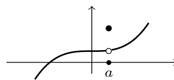
non continue en a
