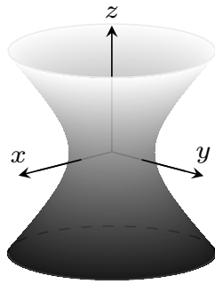
Hyperboloïde à une nappe
