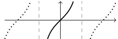
La fonction tangente restreinte à ] - \pi/2, \pi/2[ est inversible
