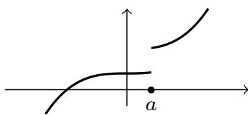
non continue en a
