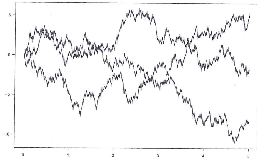
FIG. 3.1 - Trajectoires Browniennes
