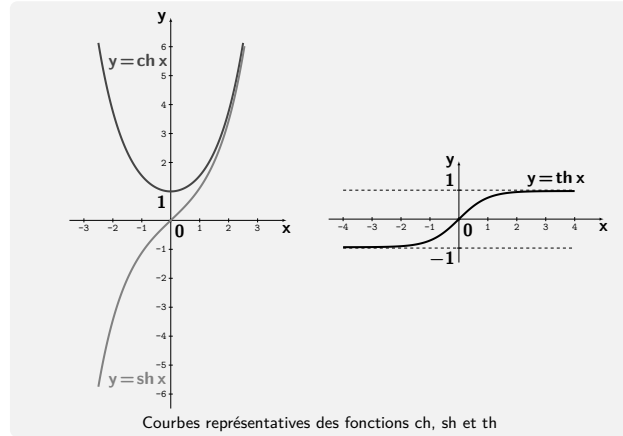
Courbes représentatives des fonctions \text{ch} , \text{sh} et \text{th}
