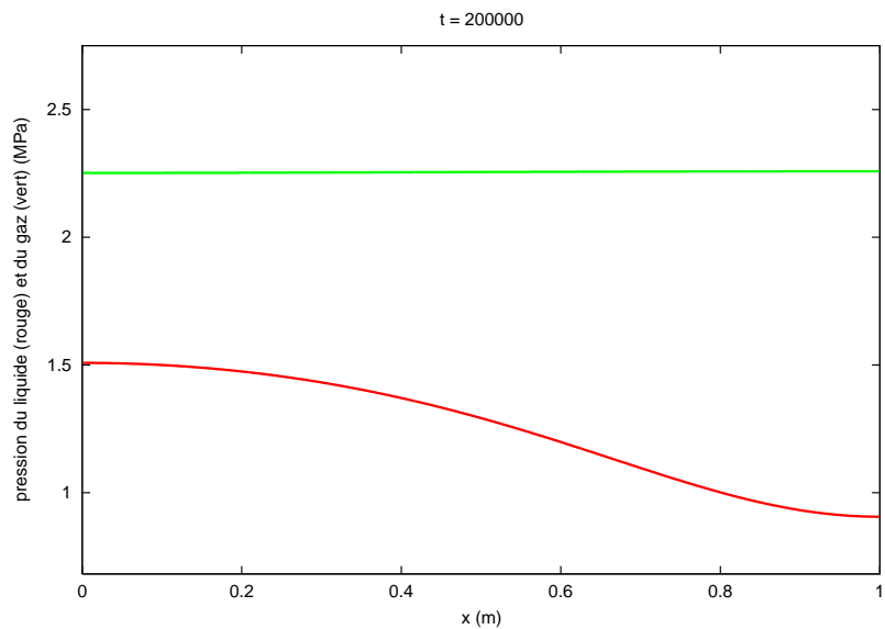
FIGURE 17 – Profil de la pression du liquide (en rouge) et du gaz (en vert) suivant l'axe x au temps t = 200000 s
