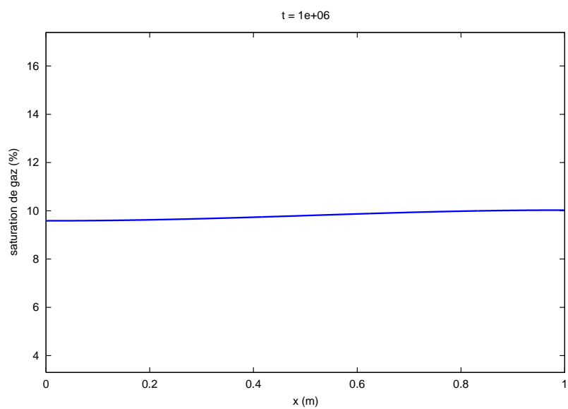
FIGURE 22 – Profil de la saturation de gaz suivant l'axe x au temps t = 1000000 s
