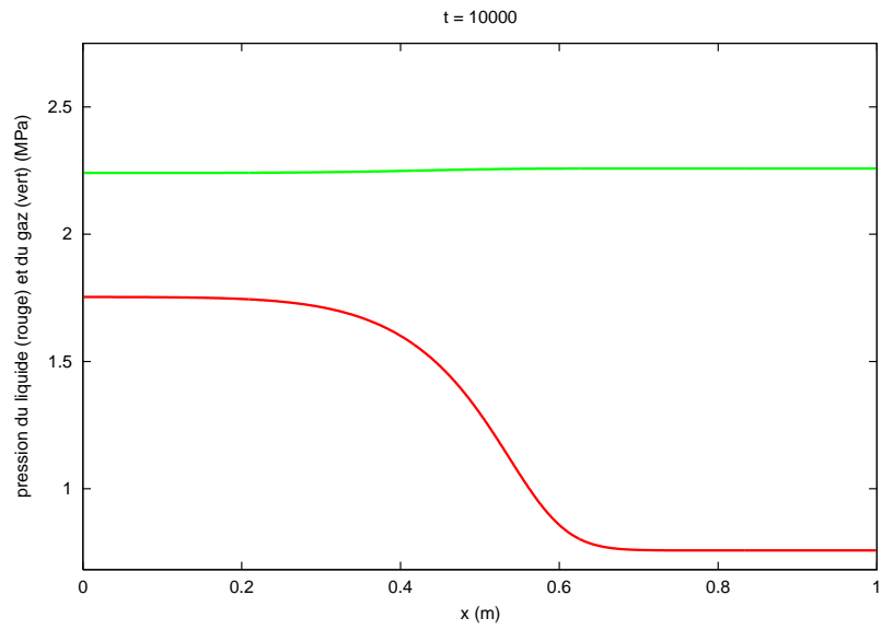
FIGURE 11 – Profil de la pression du liquide (en rouge) et du gaz (en vert) suivant l'axe x au temps t = 10000 s
