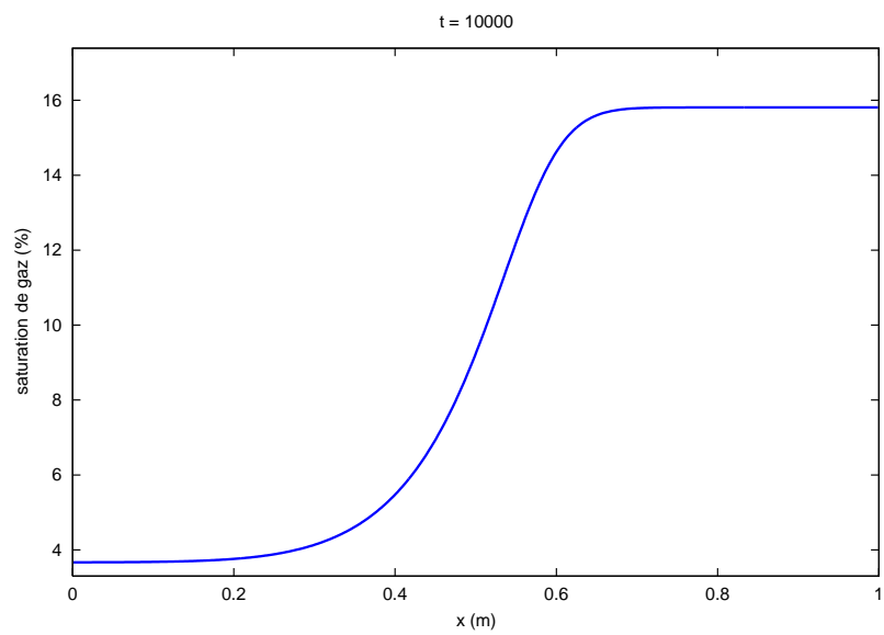
FIGURE 12 – Profil de la saturation de gaz suivant l'axe x au temps t = 10000 s
