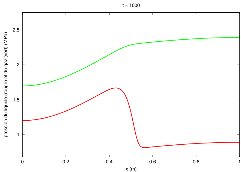
FIGURE 7 – Profil de la pression du liquide (en rouge) et du gaz (en vert) suivant l'axe x au temps t = 1000 s
