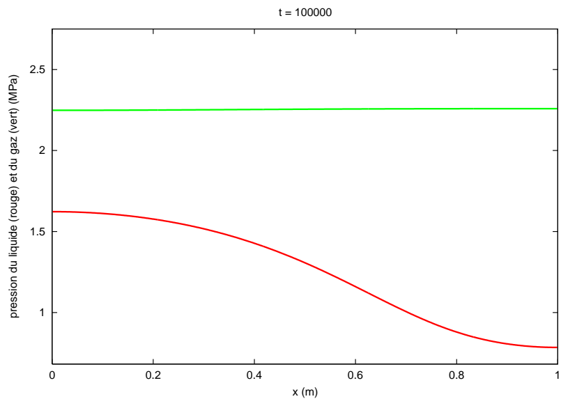
FIGURE 15 – Profil de la pression du liquide (en rouge) et du gaz (en vert) suivant l'axe x au temps t = 100000 s
