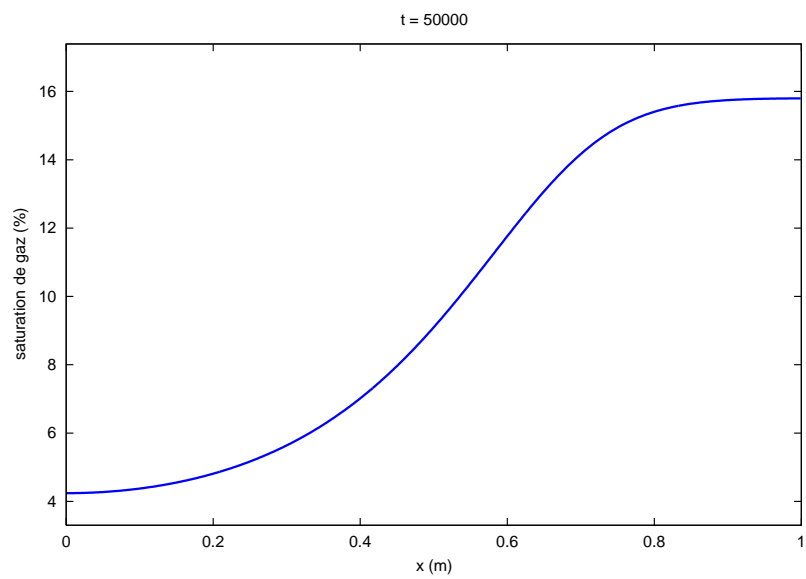
FIGURE 14 – Profil de la saturation de gaz suivant l'axe x au temps t = 50000 s
