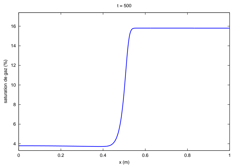
FIGURE 6 – Profil de la saturation de gaz suivant l'axe x au temps t = 500 s
