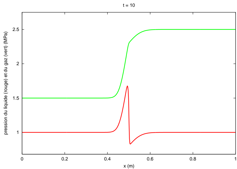
FIGURE 1 – Profil de la pression du liquide (en rouge) et du gaz (en vert) suivant l'axe x au temps t = 10 s
