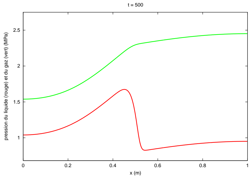
FIGURE 5 – Profil de la pression du liquide (en rouge) et du gaz (en vert) suivant l'axe x au temps t = 500 s
