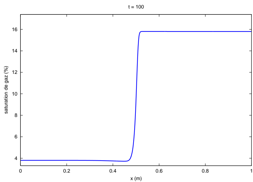
FIGURE 4 – Profil de la saturation de gaz suivant l'axe x au temps t = 100 s
