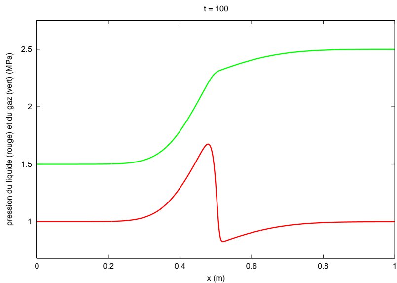
FIGURE 3 – Profil de la pression du liquide (en rouge) et du gaz (en vert) suivant l'axe x au temps t = 100 s
