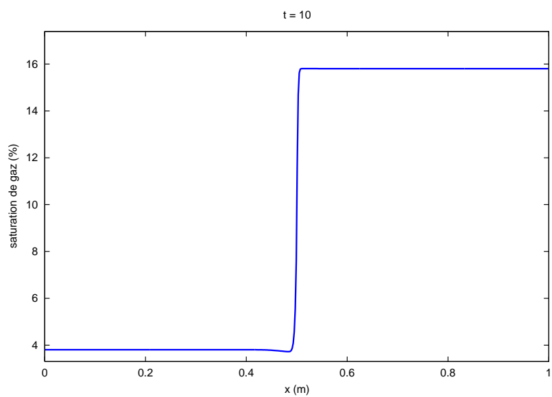
FIGURE 2 – Profil de la saturation de gaz suivant l'axe x au temps t = 10 s
