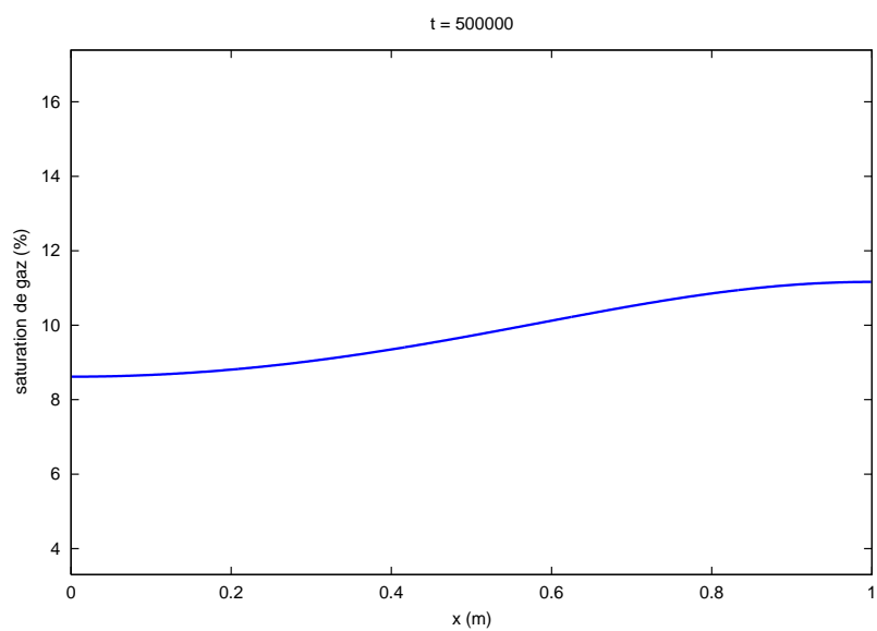
FIGURE 20 – Profil de la saturation de gaz suivant l'axe x au temps t = 500000 s
