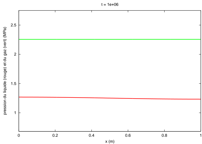
FIGURE 21 – Profil de la pression du liquide (en rouge) et du gaz (en vert) suivant l'axe x au temps t = 1000000 s
