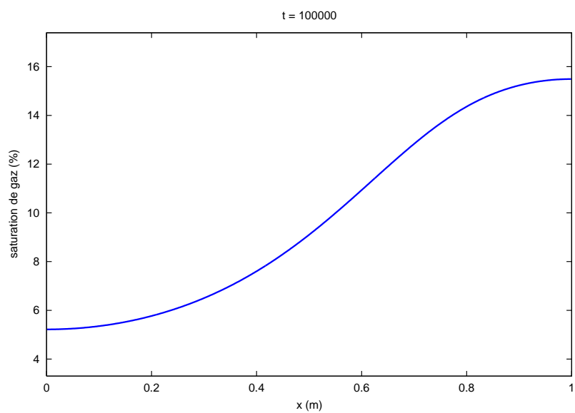
FIGURE 16 – Profil de la saturation de gaz suivant l'axe x au temps t = 100000 s
