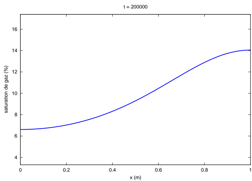
FIGURE 18 – Profil de la saturation de gaz suivant l'axe x au temps t = 200000 s
