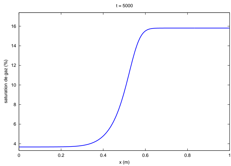
FIGURE 10 – Profil de la saturation de gaz suivant l'axe x au temps t = 5000 s
