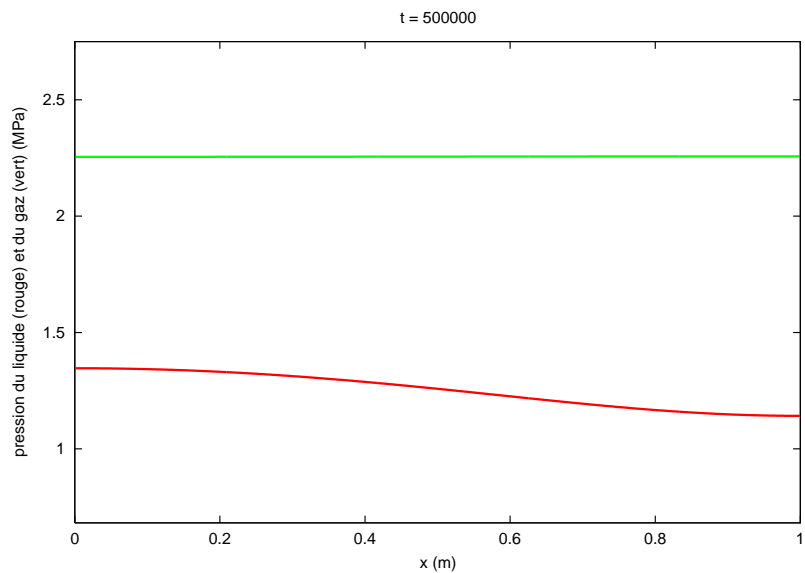
FIGURE 19 – Profil de la pression du liquide (en rouge) et du gaz (en vert) suivant l'axe x au temps t = 500000 s
