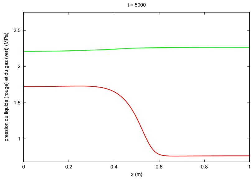
FIGURE 9 – Profil de la pression du liquide (en rouge) et du gaz (en vert) suivant l'axe x au temps t = 5000 s
