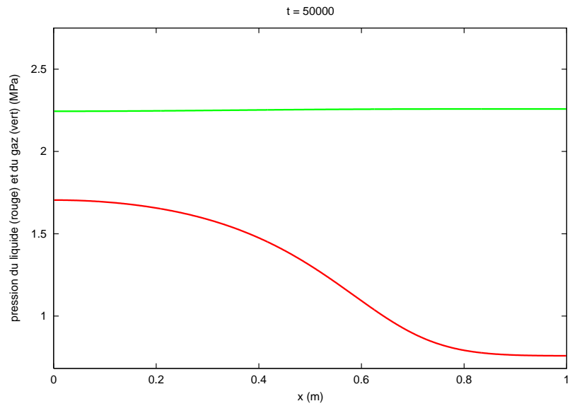
FIGURE 13 – Profil de la pression du liquide (en rouge) et du gaz (en vert) suivant l'axe x au temps t = 50000 s
