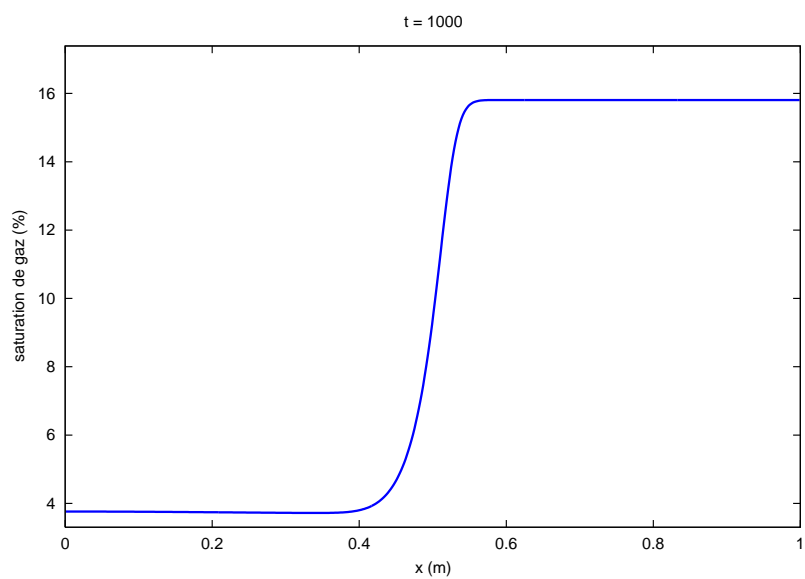
FIGURE 8 – Profil de la saturation de gaz suivant l'axe x au temps t = 1000 s
