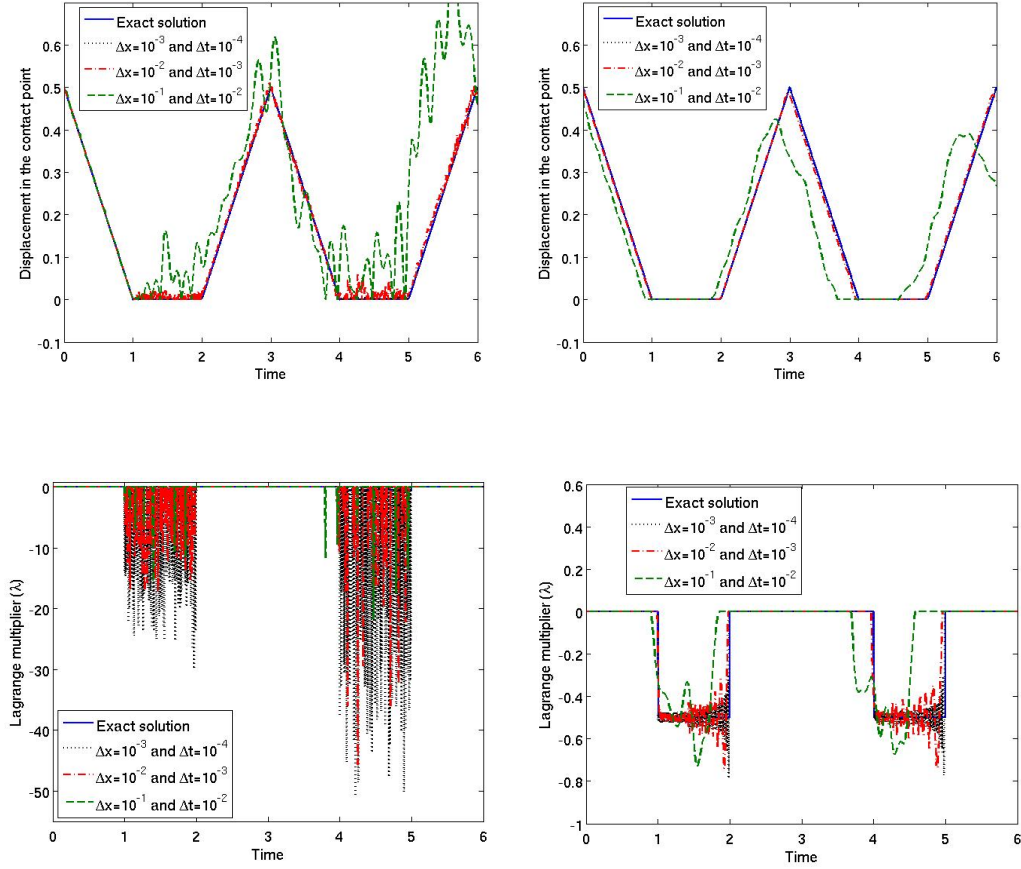
Figure 8: Comparaison de la solution analytique (u, \lambda) et des solutions approchées (U_h^n, \lambda_h^n) obtenues en utilisant les matrices de masse standard (à gauche) et modifiée (à droite) au nœud de contact.
