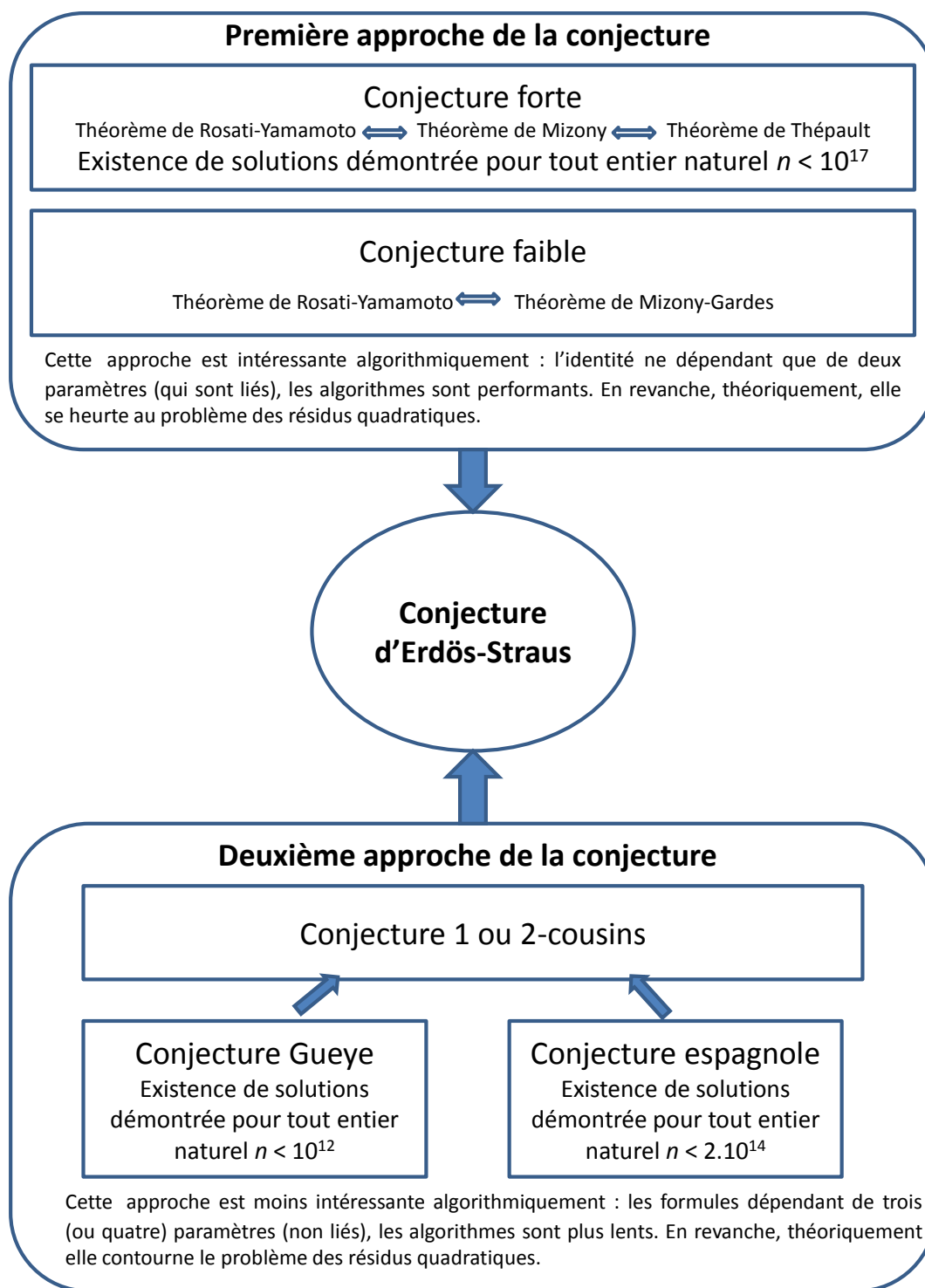
FIGURE 1 – Un bilan sur les différentes conjectures énoncées
