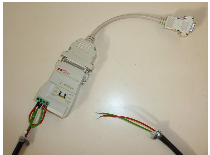
Adaptateur + câble monté (Le bloc adaptateur d'alimentation secteur n'apparaît pas ici, mais ne l'oubliez pas !)
