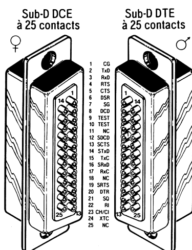
Canon Sub-D 25 broches
