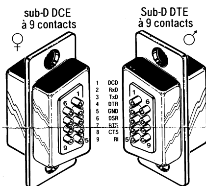
Canon Sub-D 9 broches
