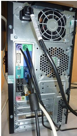
Connectique ordinateur PC avec port série 9 broches
